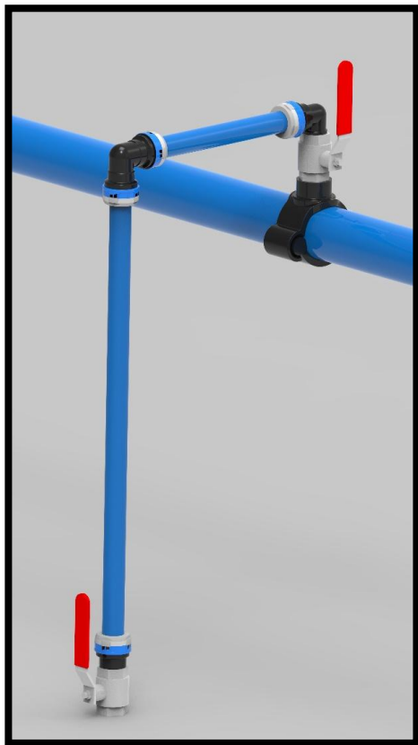
Vista Isométrica
